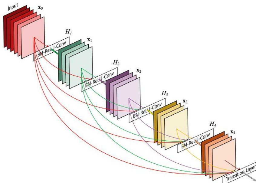
Hình 1.1. Minh họa kiến trúc DenseNet [7]
