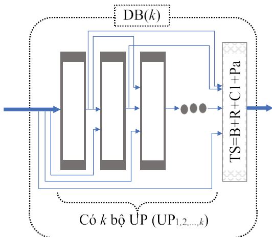
Hình 2.2. Sơ đồ kết nối trong khối DB(k)
