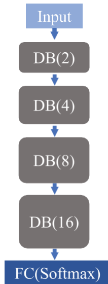
Hình 2.3. Sơ đồ các khối DB của LDFER
